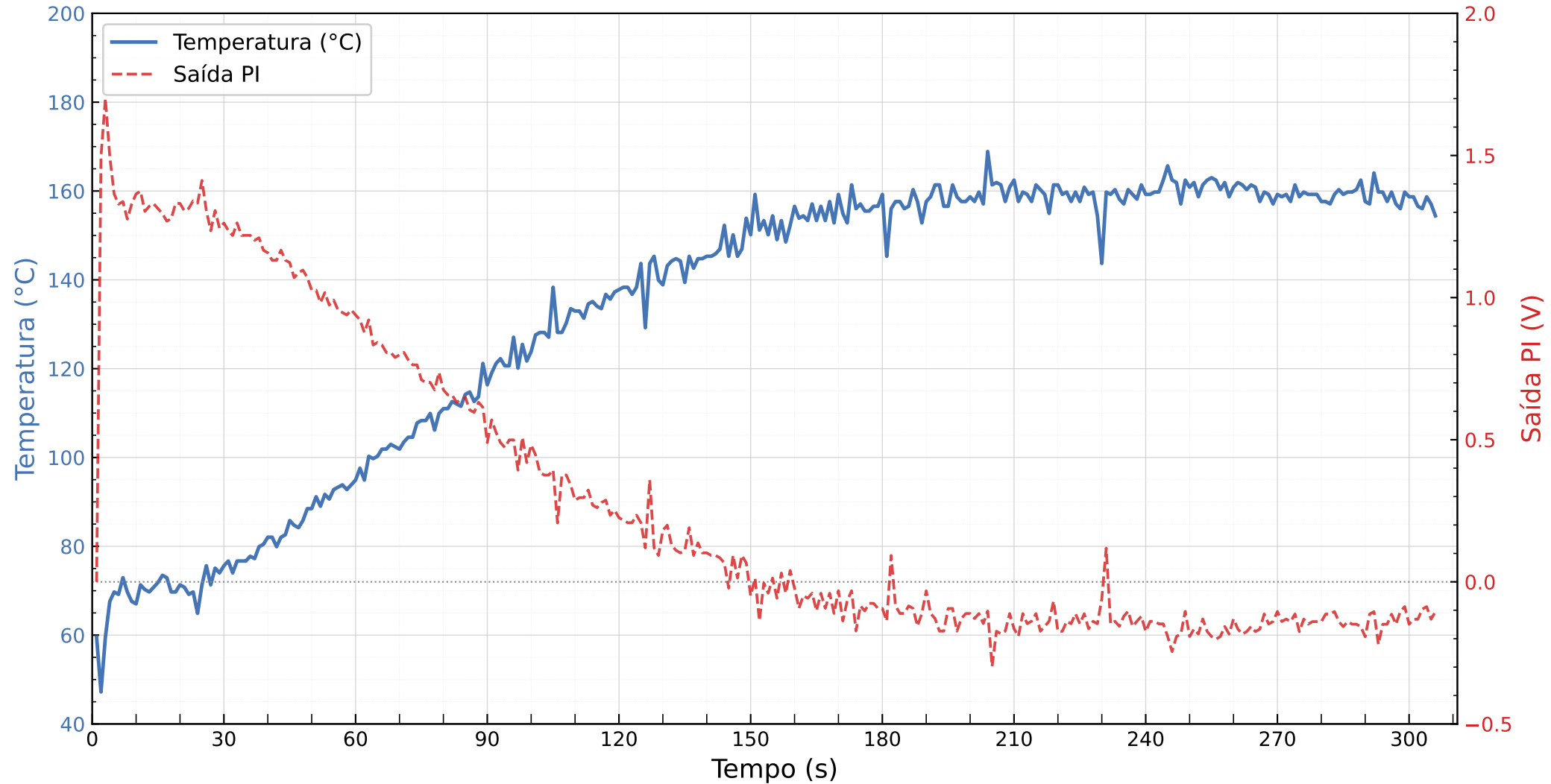
Controle PI — Resposta de Temperatura e Saída do Controlador
